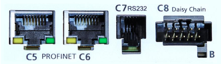
图 11-2 PROFINET 机型上的上面板接口和 LED
