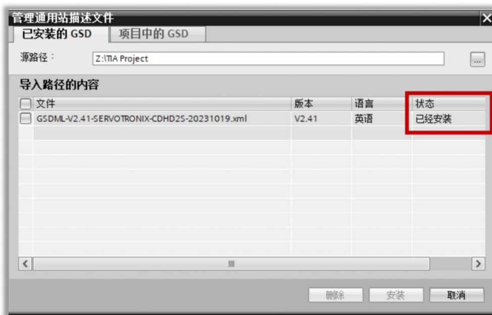
图 9-11 确认 GSD 文件状态为已经安装
