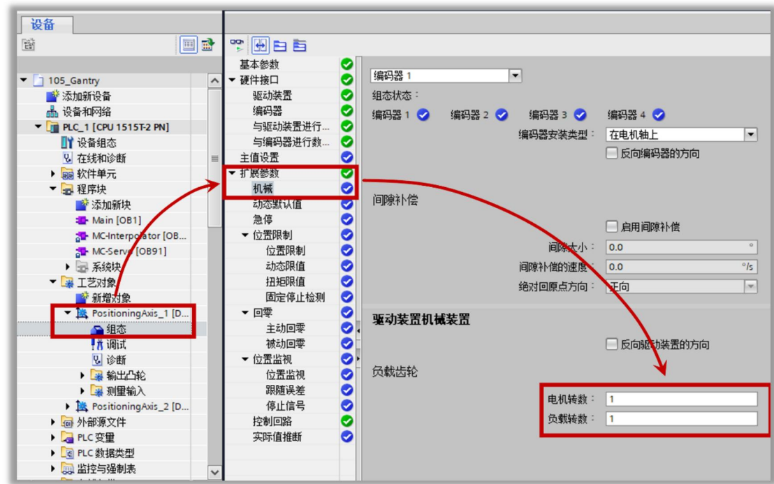
图 9-39 工艺对象中机械参数的设置
