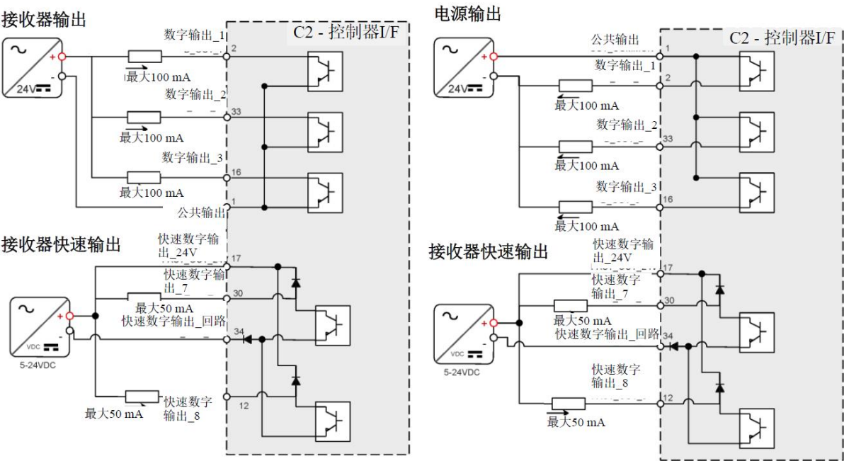
图 4-18 数字输出接线 - C2
