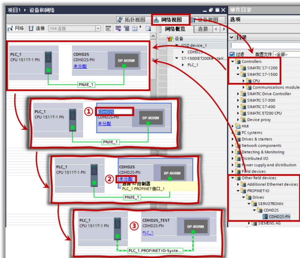
图 9-12 添加 PLC 和高创 CDHD2S
