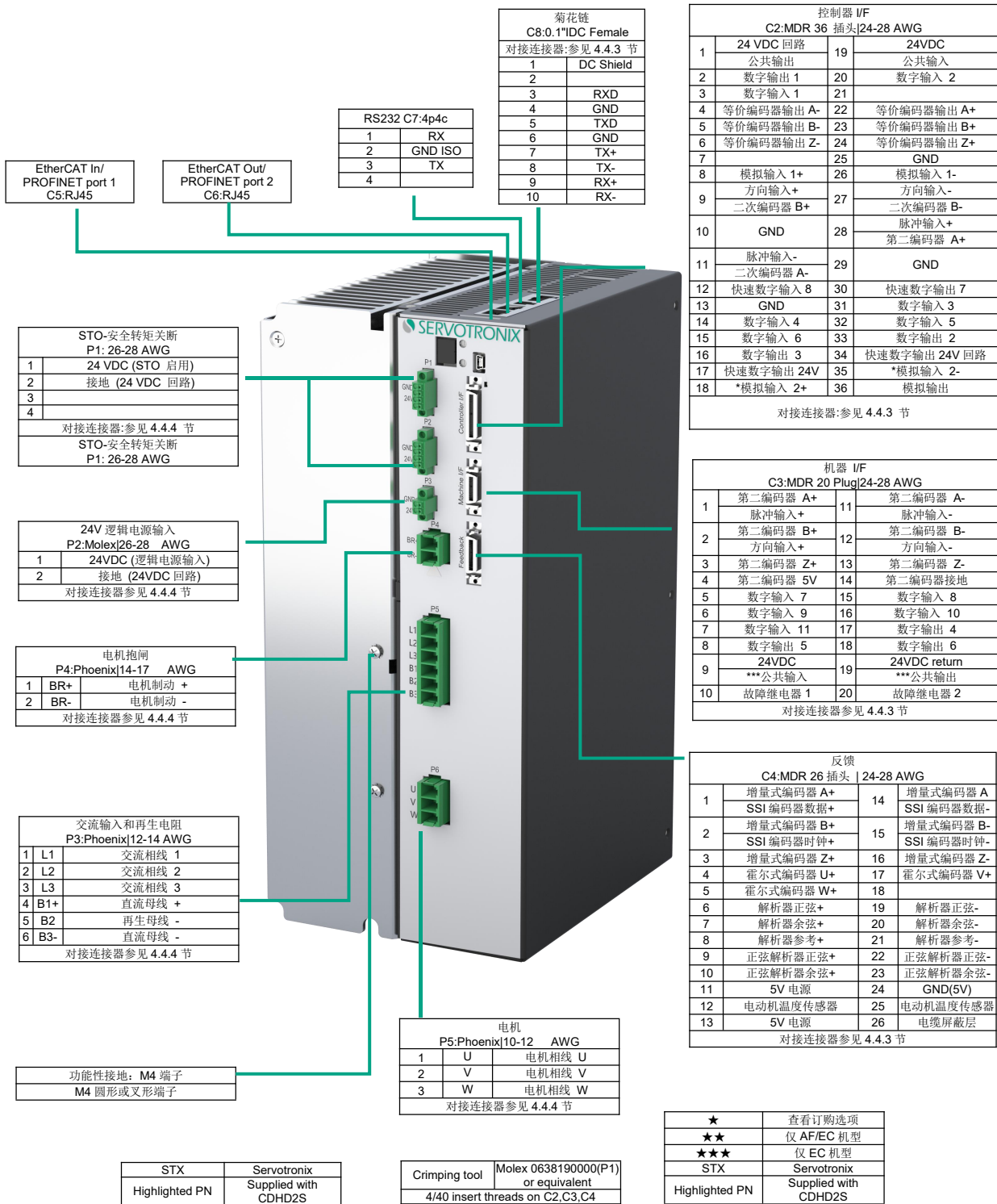
图 4-34 CDHD2S-024/CDHD2S-030 (高压) 功率板引脚分配
