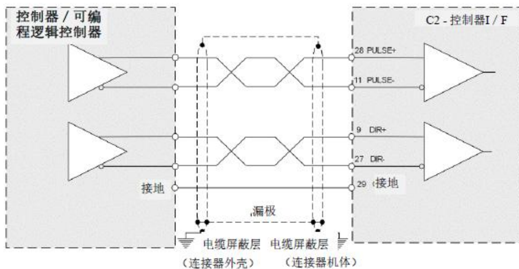
图 4-22 脉冲和方向光学隔离输入接线 - C2
