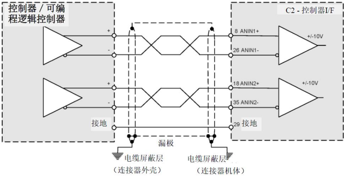
图 4-19 模拟输入接线-C2
