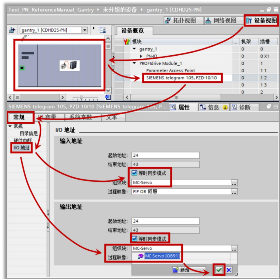
图 9-30 驱动器报文的组织块设置
