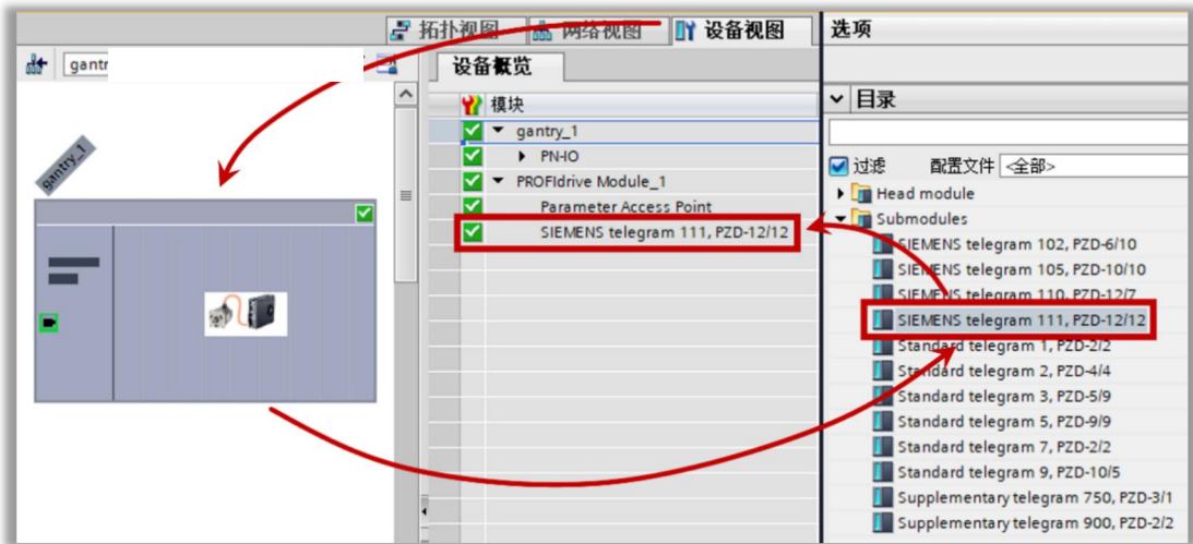
图 9-13 为驱动器添加 111 报文
