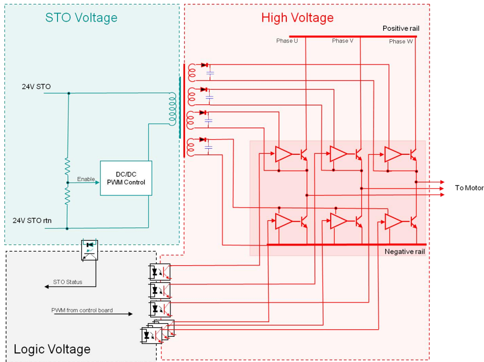
图 10-2 STO 电路结构
