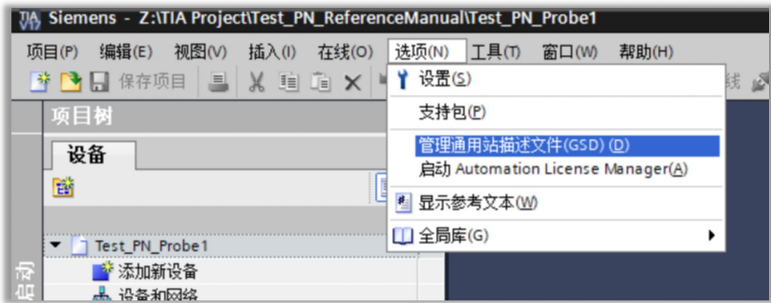
图 9-10 安装 GSD 文件
