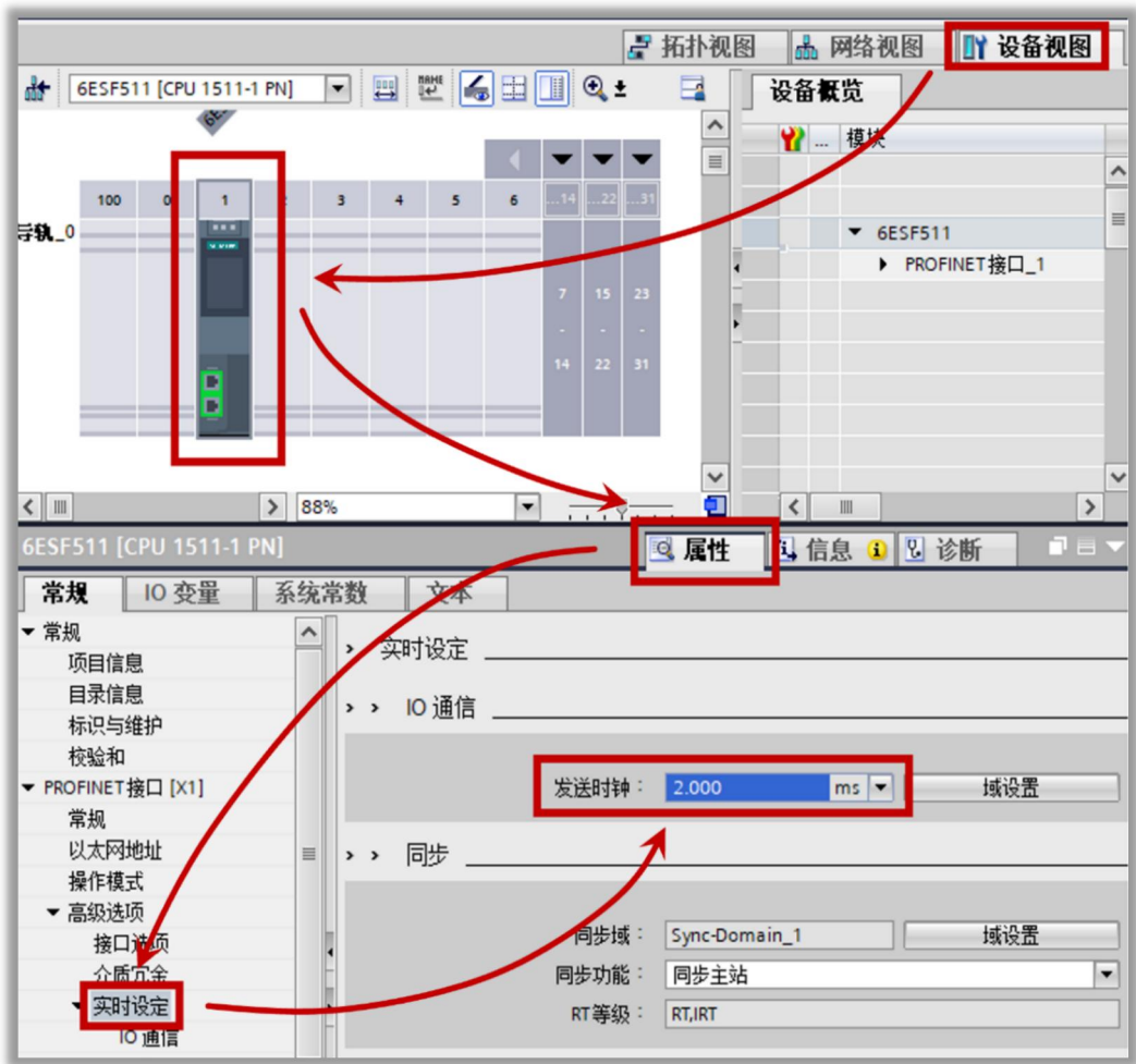
图 9-28 组态设置 PLC 发送时钟设置
