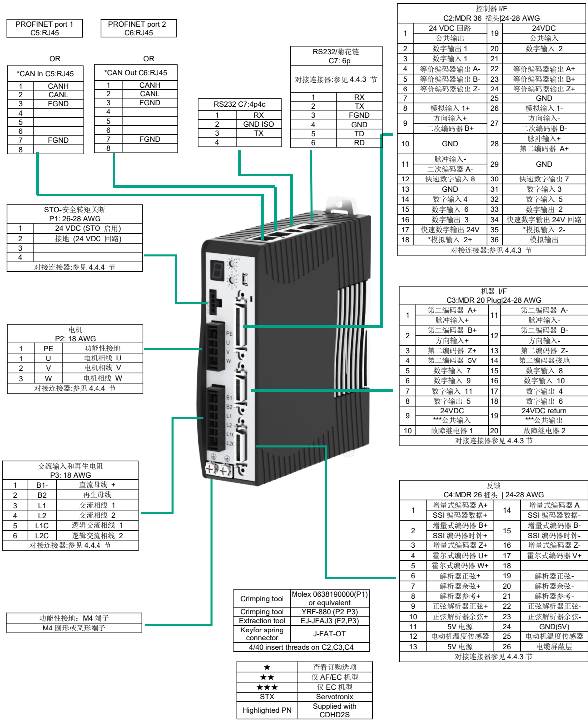
图 4-29 CDHD2S-1D5/003(中压 PN)功率板引脚分配
