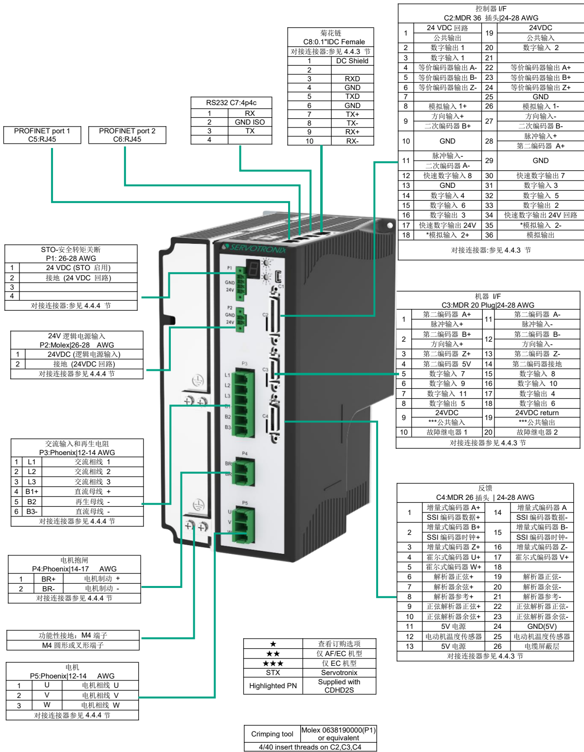
图 4-33 CDHD2S-012(高压) 功率板引脚分配
