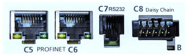
图 9-1 CDHD2S-PN 顶部面板的接口
