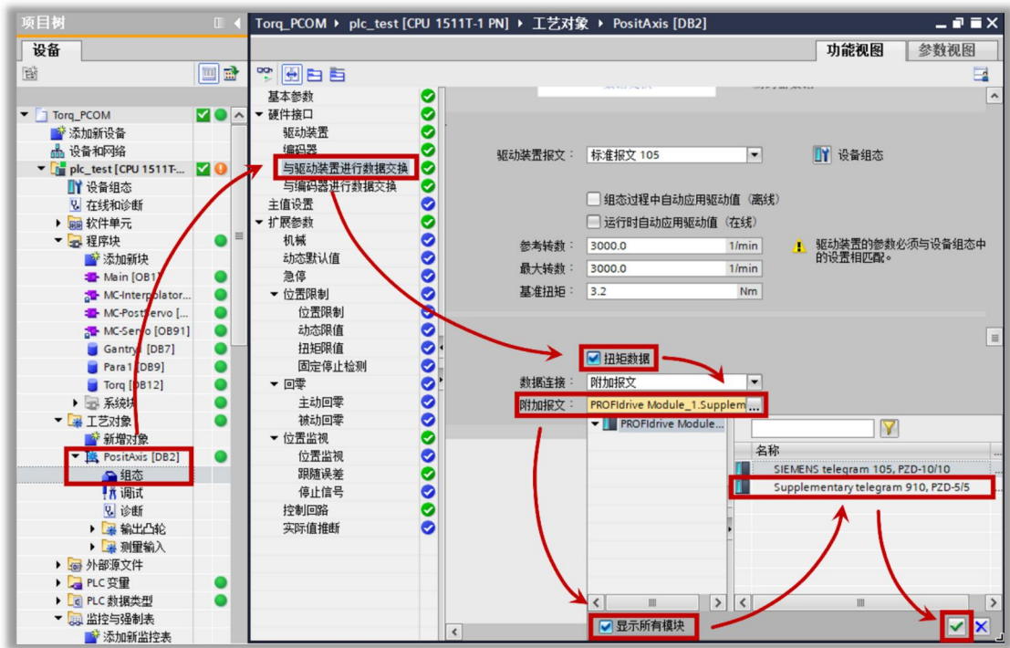
图 9-46 工艺对象中添加扭矩数据-附加报文 910
