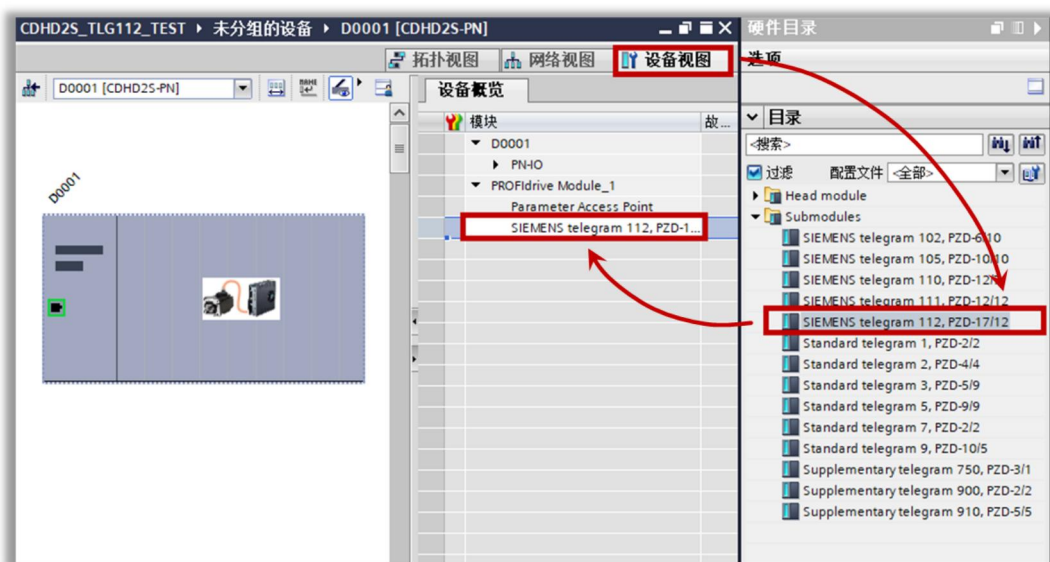
图 9-18 为驱动器添加西门子 112 报文
