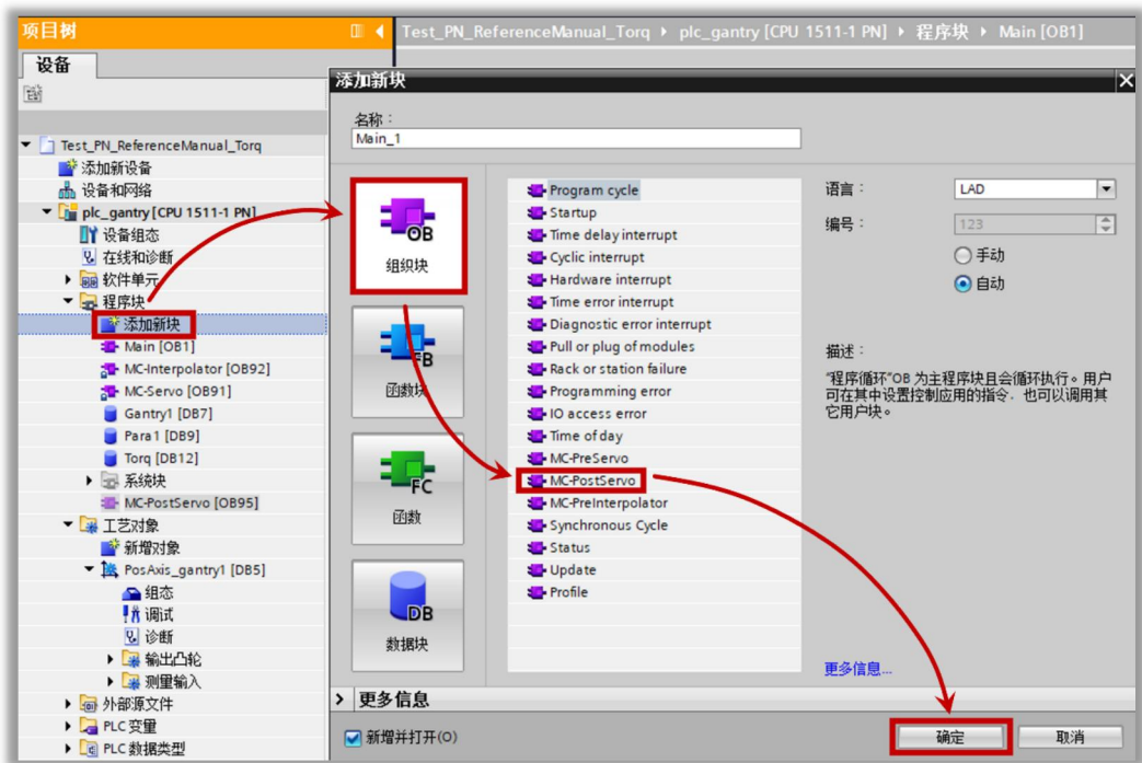
图 9-48 添加 MC_PostServo 组织块
