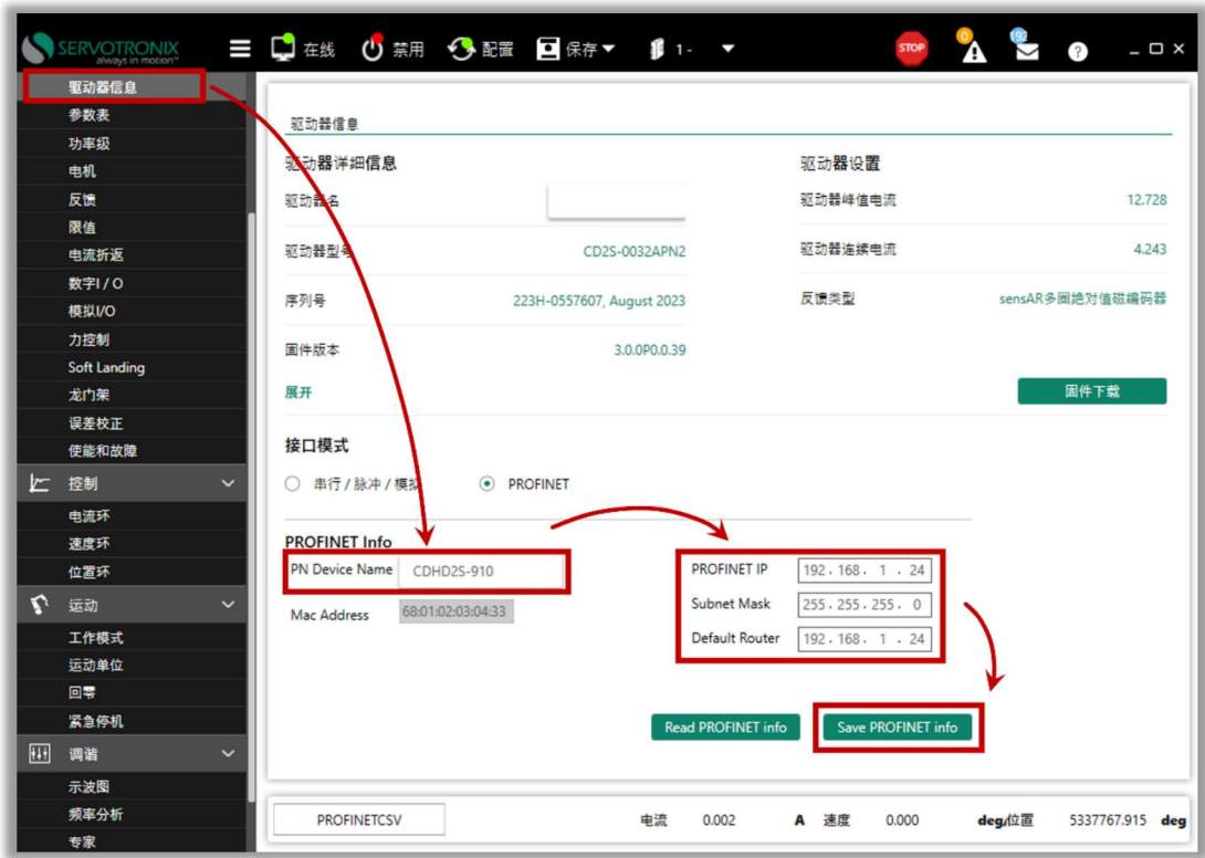
图 9-8 在 Servostudio 中设置 PROFINET IO 的 IP 和设备名
