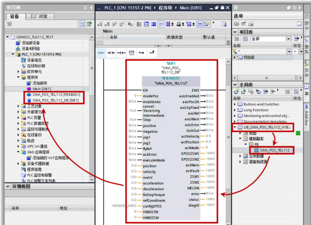
图 9-20 在程序块中添加[FB38051]功能块
