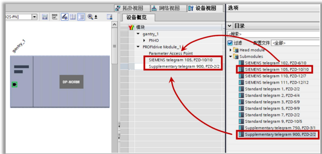
图 9-53 为驱动器配置 105 和 900 报文
