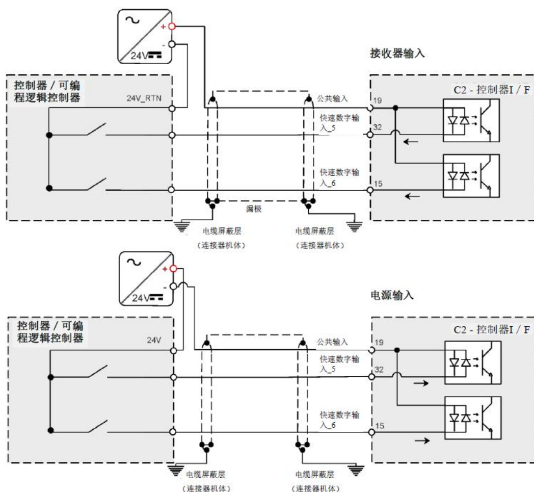
图 4-21 脉冲和方向光学隔离输入接线-C2
