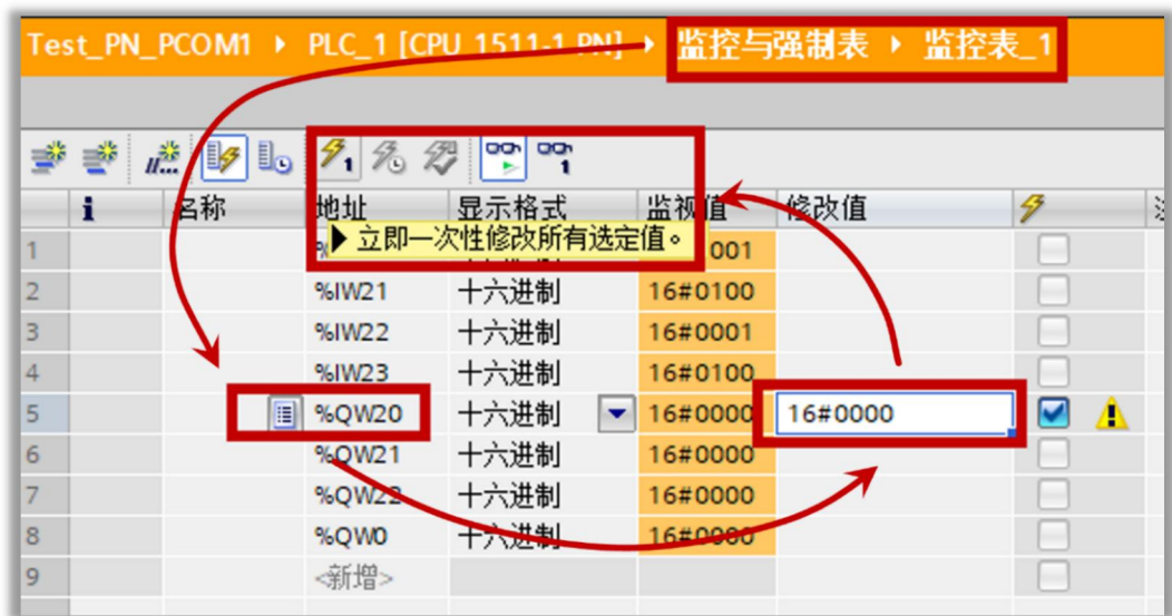
图 9-54 修改 PCOM1 控制字
