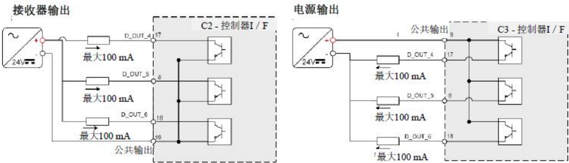
图 4-25 数字输出接线 - C3
