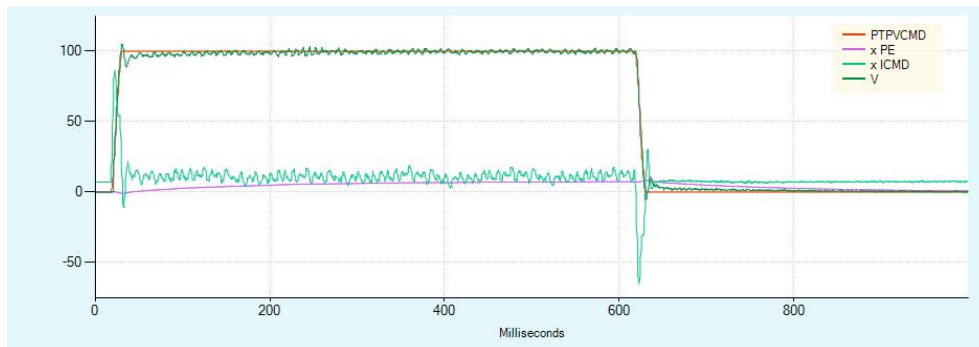
图 8-43 双反馈—调谐位置控制器 (KNLDUALLOOPVFF) 一示例
