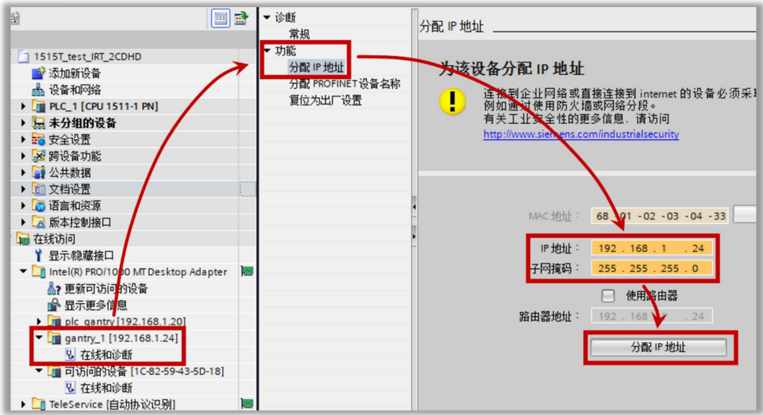
图 9-5 为驱动器分配 IP 地址
