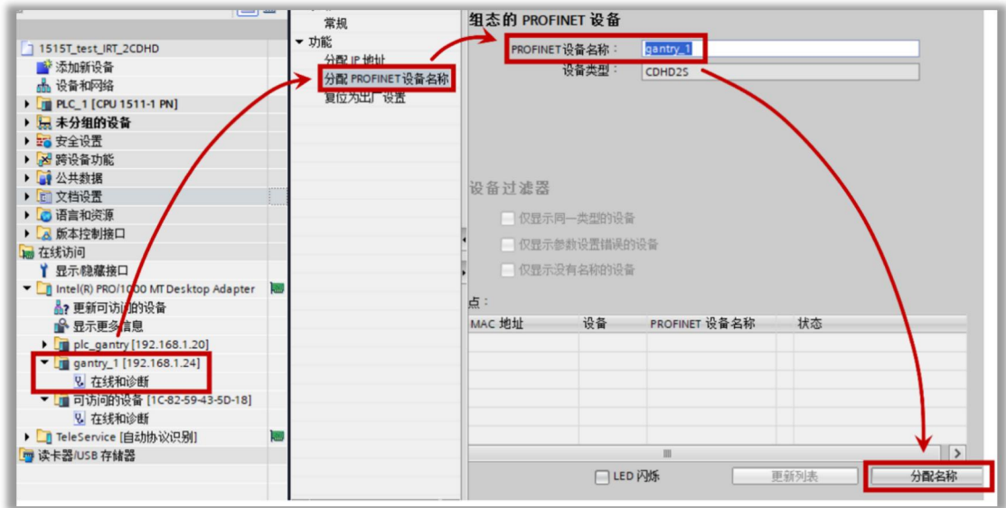
图 9-7 为驱动器分配设备名
