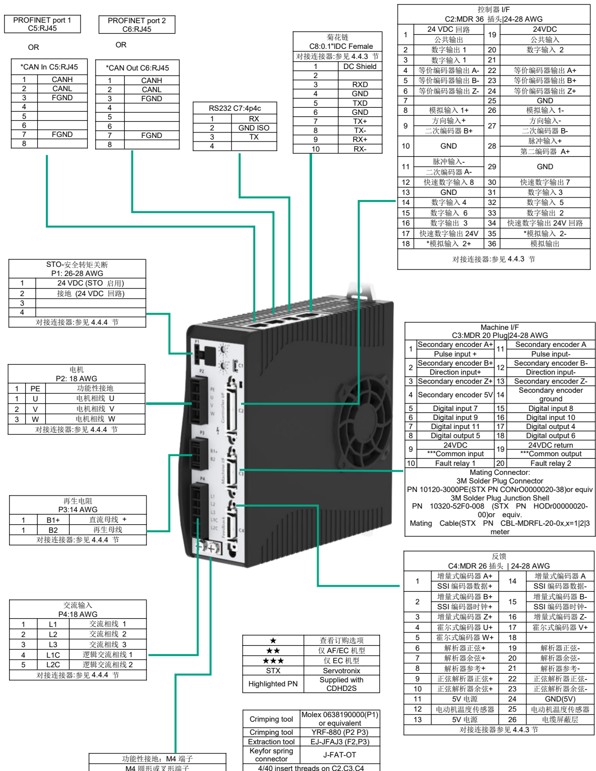
图 4-30 CDHD2S-4D5/006(中压 PN 型号)功率板引脚分配
