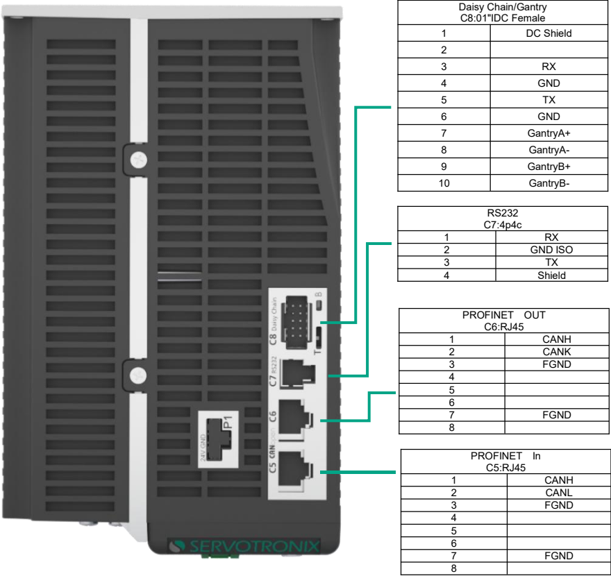
图 4-16 CDHD2S PN 型号上面板引脚分配
