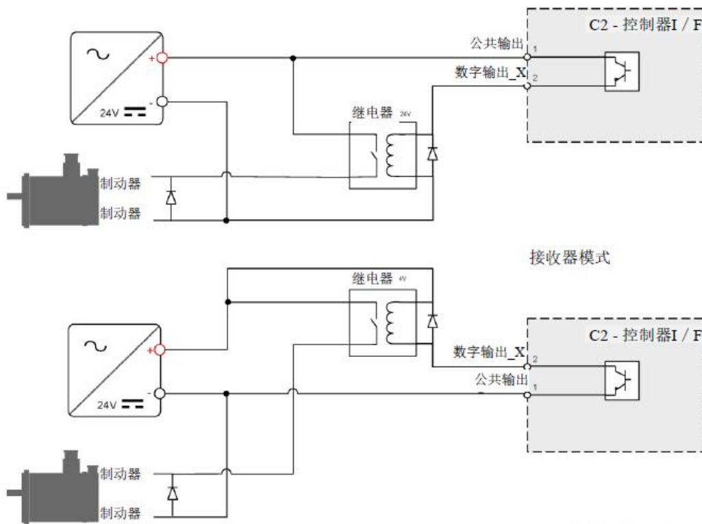
图 4-26 电机制动器接线 CDHD2S (中压型号)
