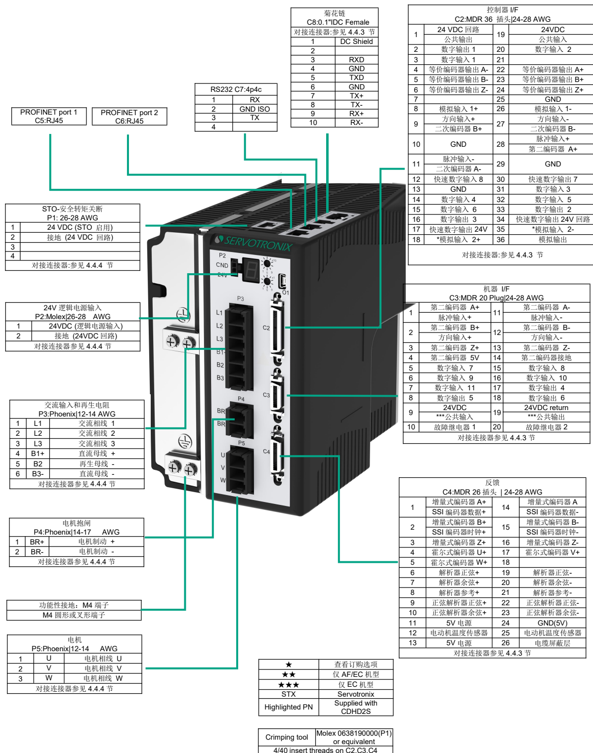
图 4-32 CDHD2S-003/CDHD2S-006(高压)功率板引脚分配
