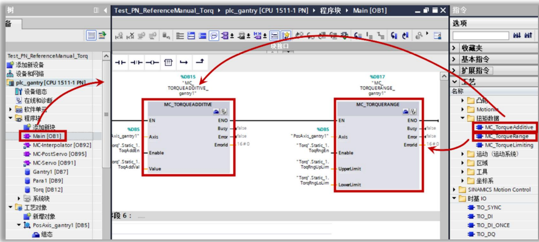
图 9-50 添加 MC_TORQUEADDITIVE 和 MC_TORQUEANGE 组织块
