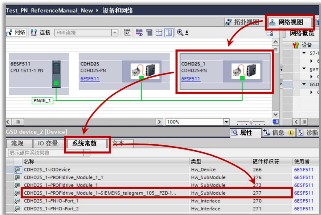
图 9-51 查找驱动器报文硬件标识符
