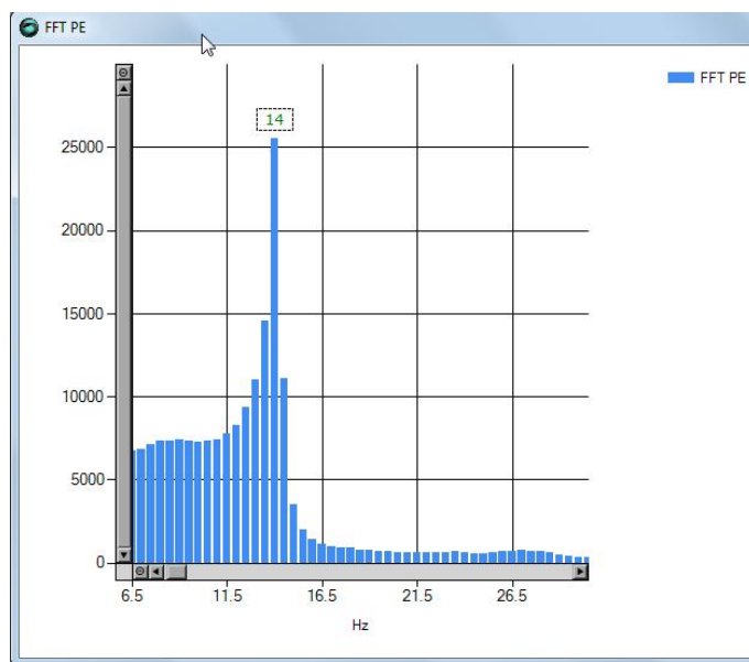
图 8-27 FFT 跟踪
