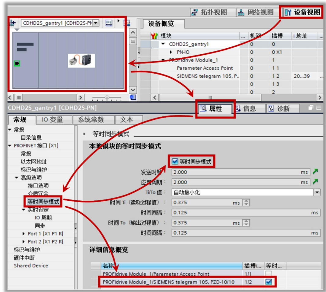
图 9-26 驱动器等时同步模式设置
