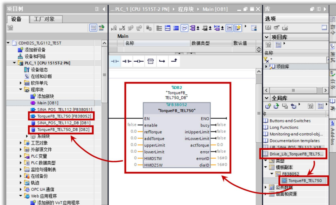
图 9-23 在程序块中添加[FB38051]功能块
