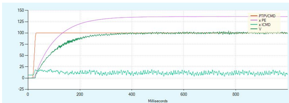
图 8-42 双反馈—调谐位置控制器 (KNLDUALLOOPKP) 一示例
