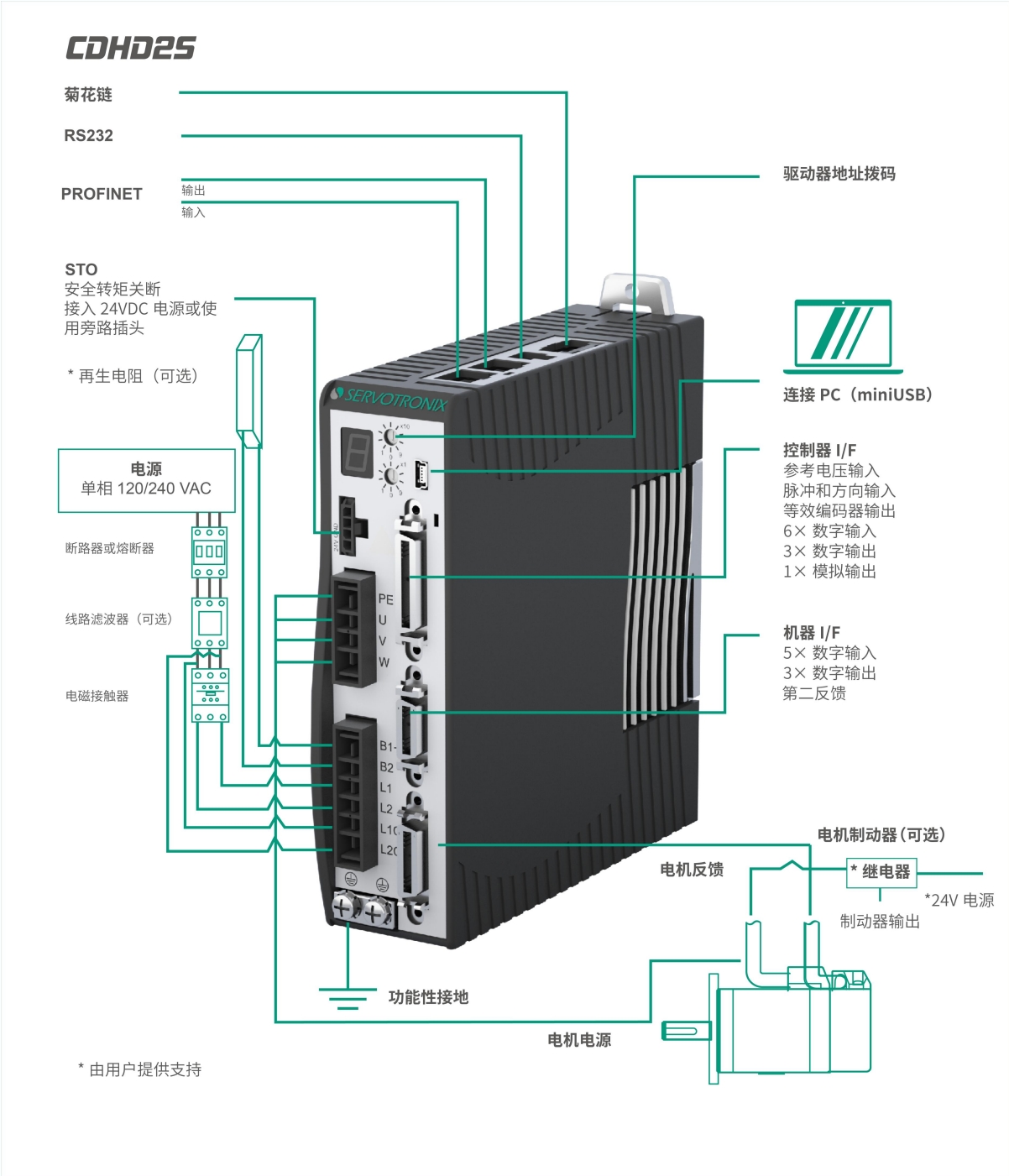
图 4-3 CDHD2S-1D5/CDHD2S-003 交流 120-240V(中压 PN)型号系统接线
