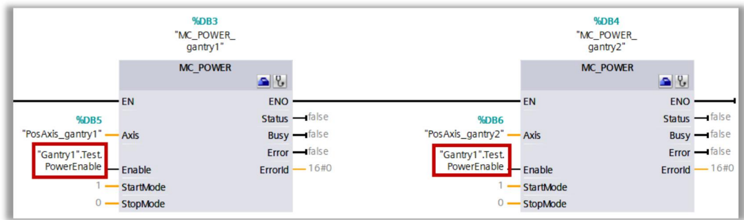
图 9-42 程序块同时使能龙门
