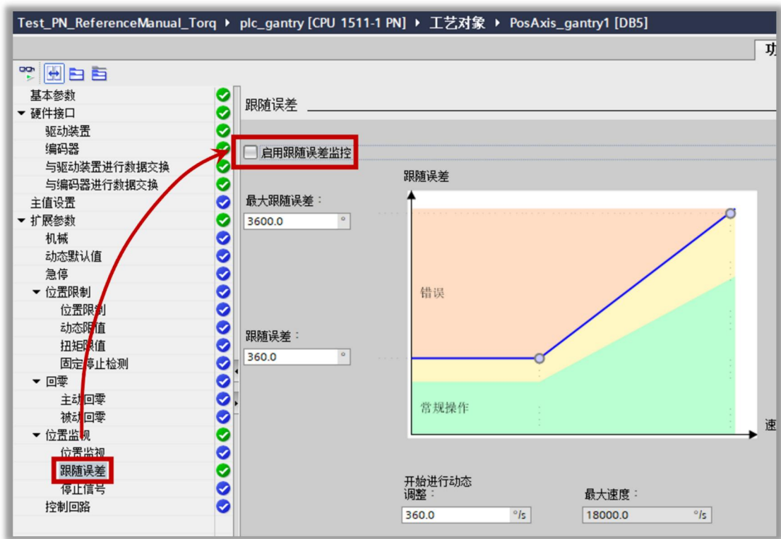
图 9-47 取消勾选启用跟随误差监控
