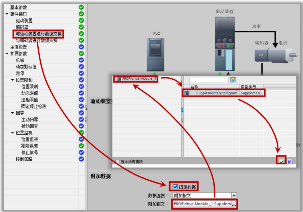
图 9-45 工艺对象中添加扭矩数据
