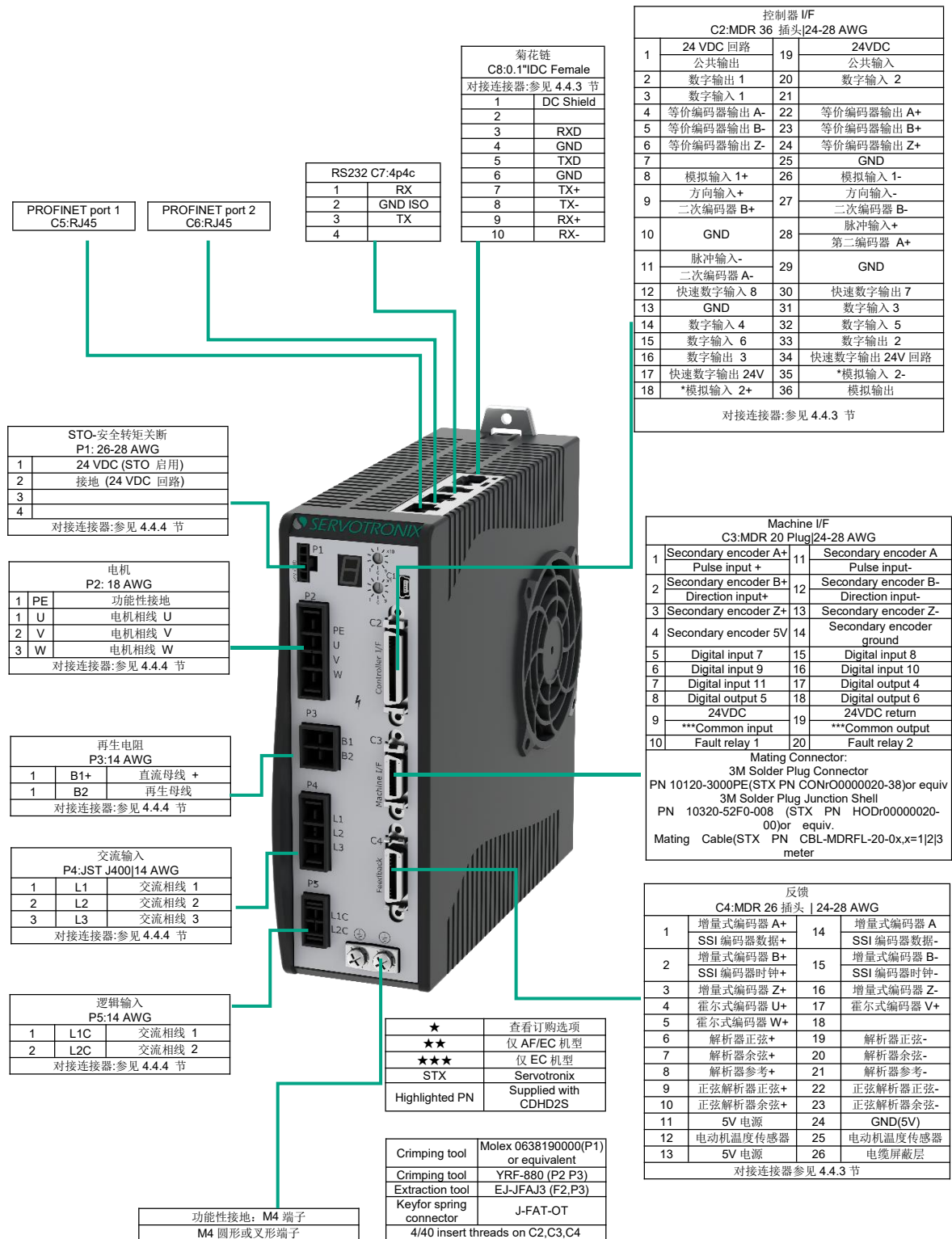
图 4-31 CDHD2S-008/010/013(中压 PN 型号)功率板引脚分配
