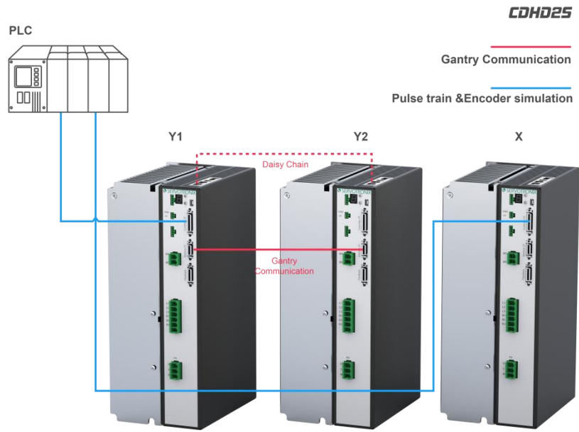
图 4-27 龙门系统接线 - 脉冲方向和串行
