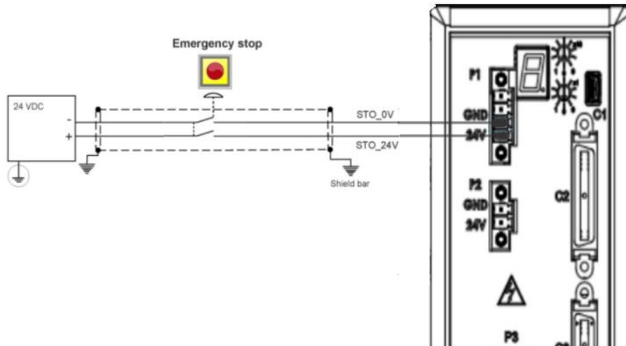
图 4-37 STO-紧急停止电路接线-示例
