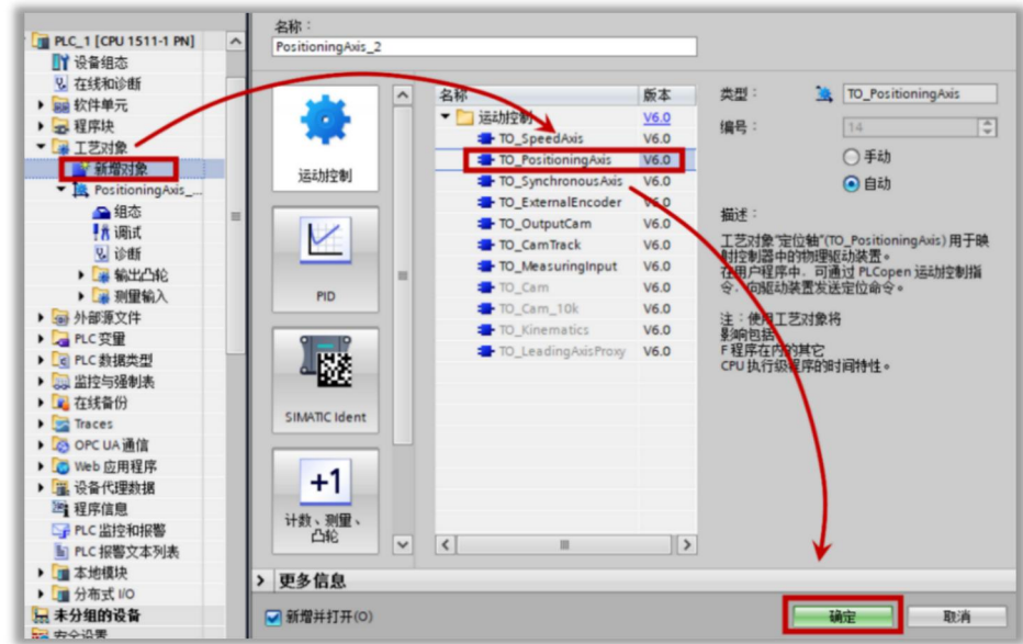
图 9-31 新增工艺对象
