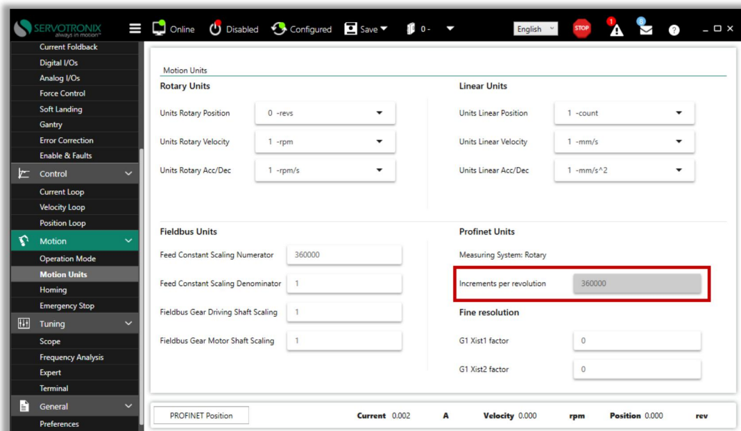
图 9-37 Servostudio 中 PROFINET 编码器数据
