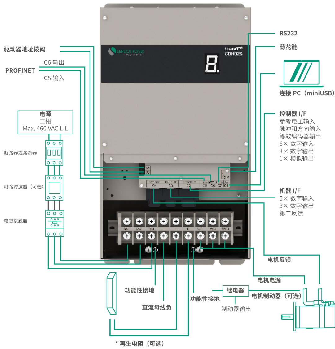
图 4-10 CDHD2S-060 交流 380V-460V (高压 PN) 型号系统接线
