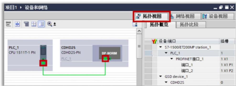
图 9-24 拓扑视图连线
