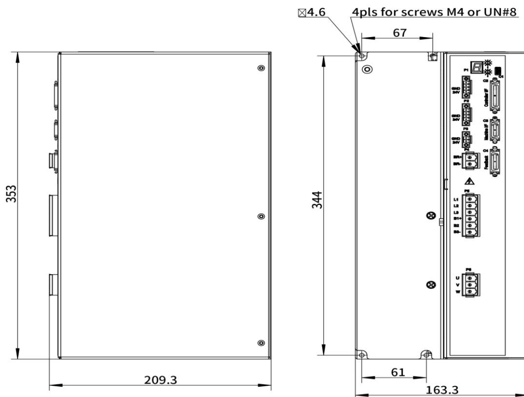
图 3-7 CDHD2S-024/CDHD2S-030(高压) - 尺寸(mm)
