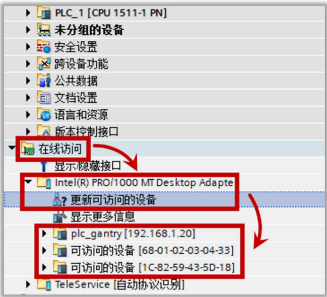
图 9-4 两在线扫描可用设备
