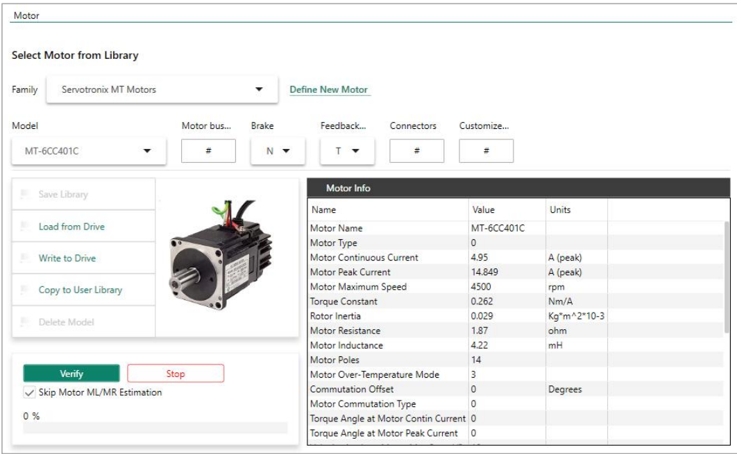
图 5-4 电机设置向导—电机选择
