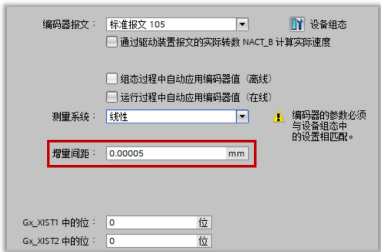
图 9-38 应用直线电机时与编码器进行数据交换的设置
