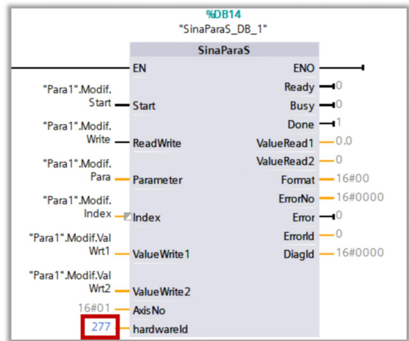
图 9-52 SinaParaS 中的 hardwareid
