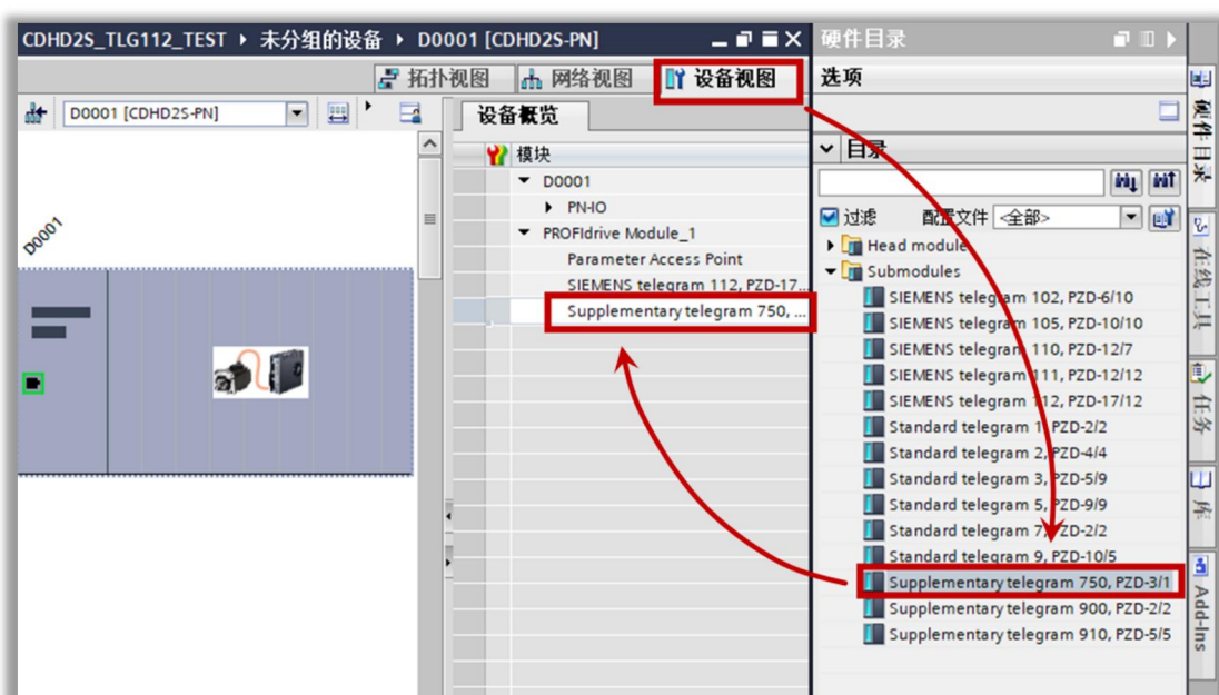
图 9-21 为驱动器添加 750 附加报文
