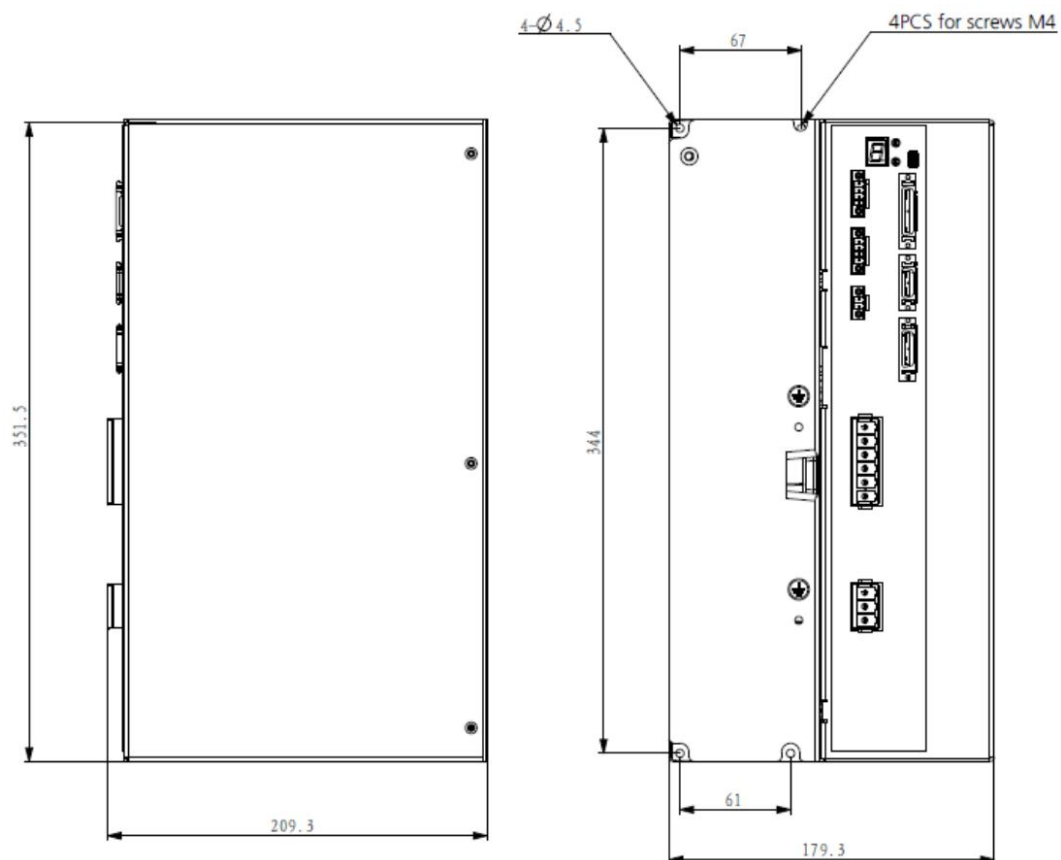
图 3-8 CDHD2S-040(高压) - 尺寸(mm)
