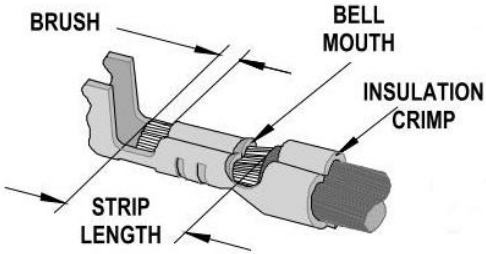
图 4-2 导线插入压接引脚
