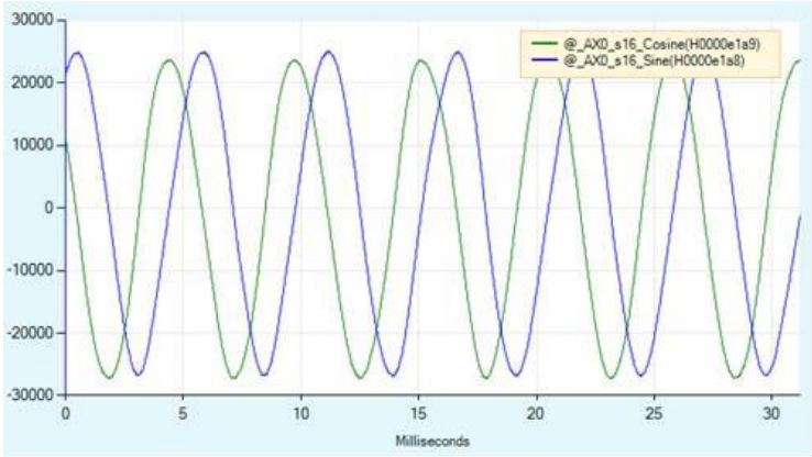
图 6-18 正弦编码器记录一示例
