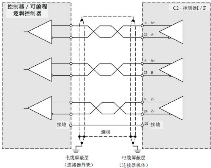
图 4-23 模拟编码器等效输出接线 - C2
