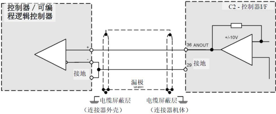
图 4-20 模拟输出接线 - C2
