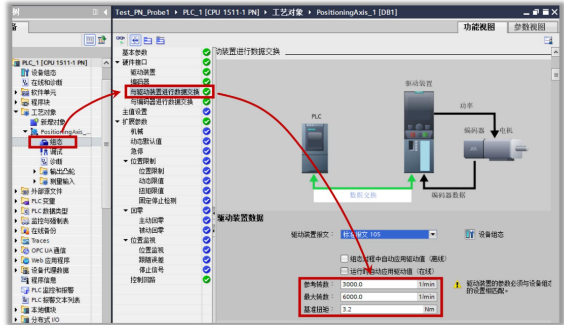
图 9-35 与驱动器进行数据交换设置
