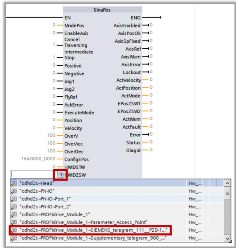
图 9-15 添加硬件标识符 ID
