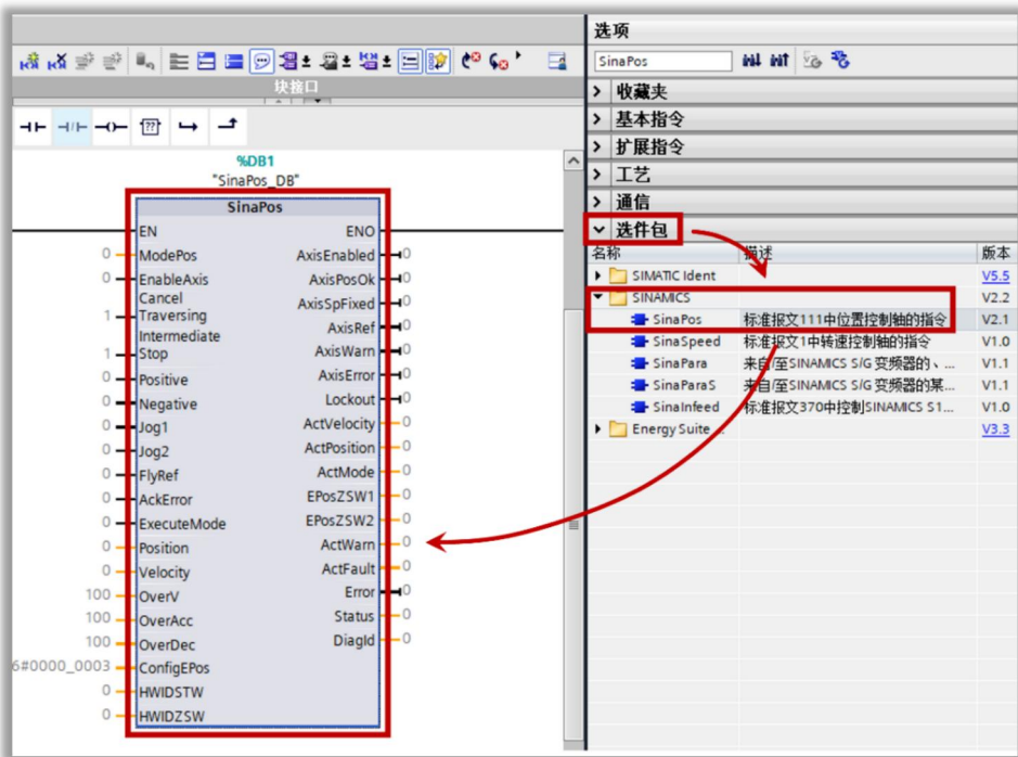
图 9-14 添加 SinaPos (FB284) 功能块
