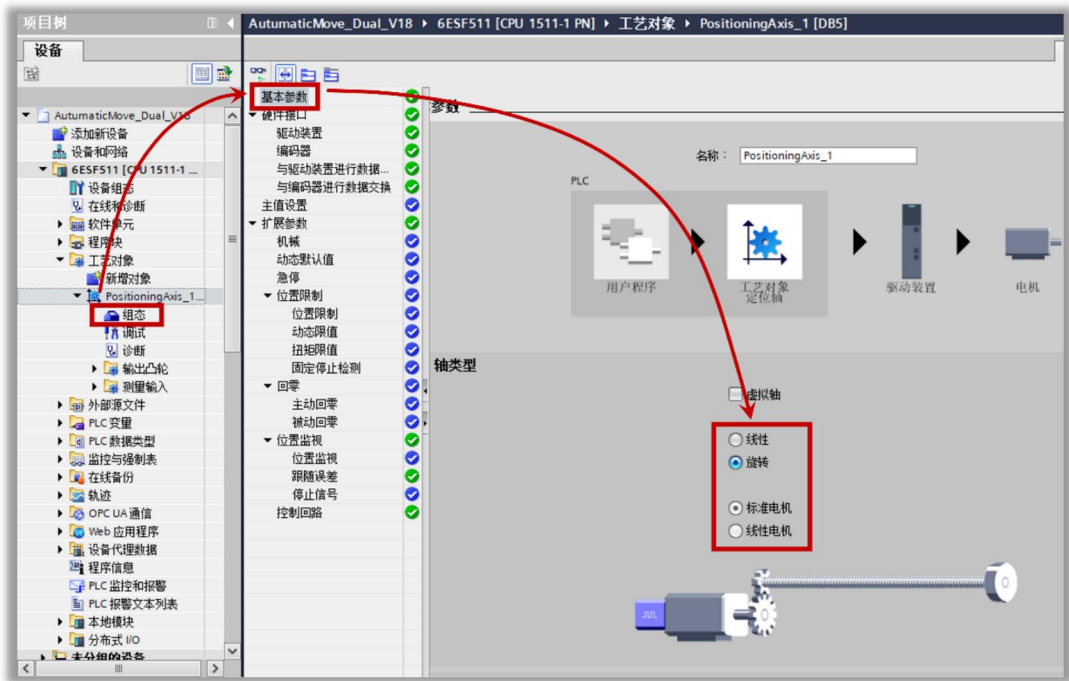
图 9-32 工艺对象组态设置
