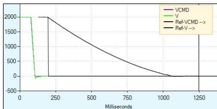
图 10-3 当 STO 生效时电机滑行停止
