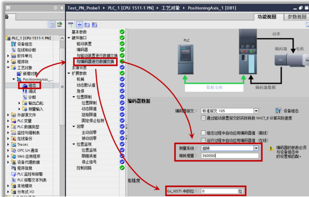
图 9-36 应用旋转电机时与编码器进行数据交换的设置
