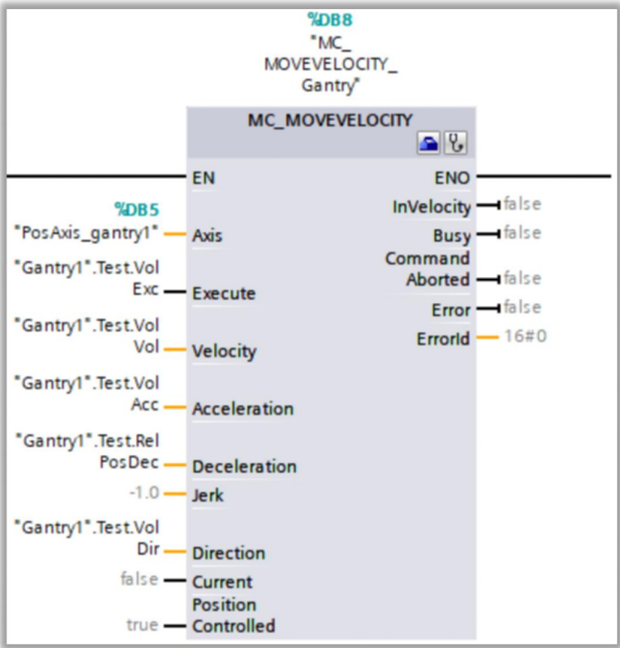
图 9-43 使用速度控制模块运行龙门
