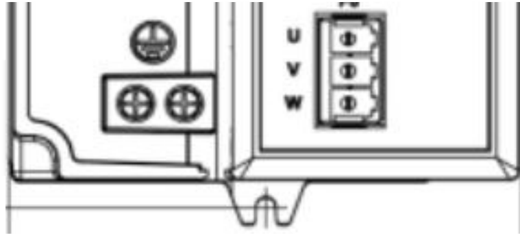
图 4-38 接地端子
