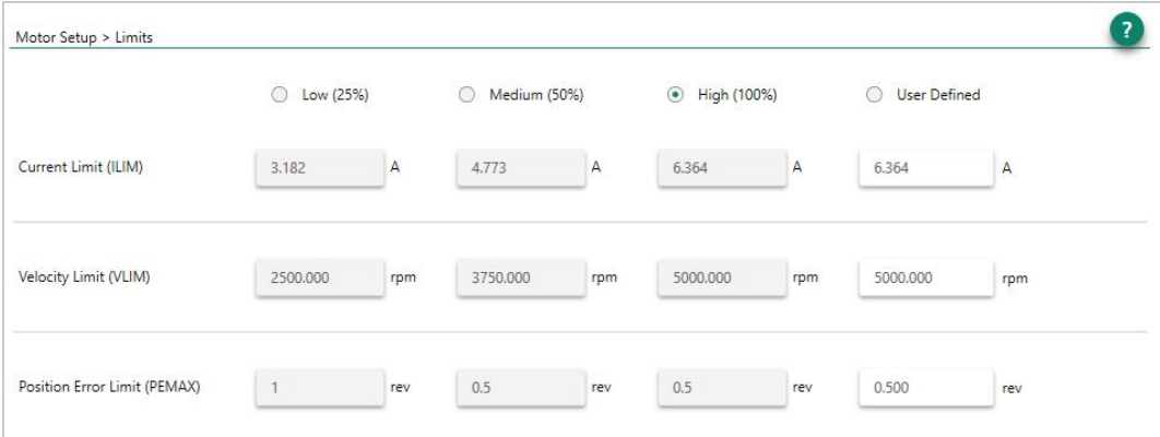
图 5-5 电机设置向导——极限
