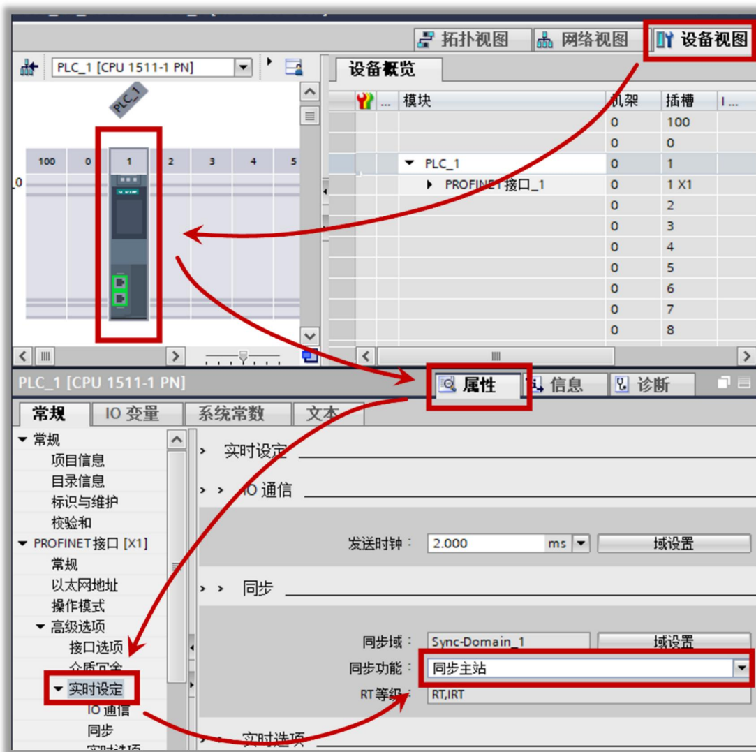
图 9-27 PLC 等时同步设置
