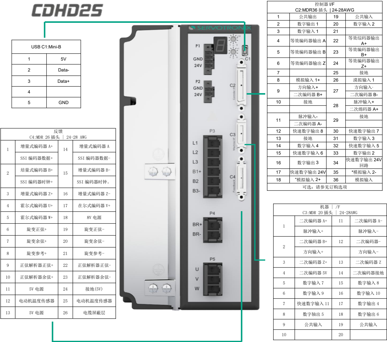
图 4-15 CDHD2S-3A/6A/12A/24A/30A/40A/60A 高压 型号控制板引脚分配
